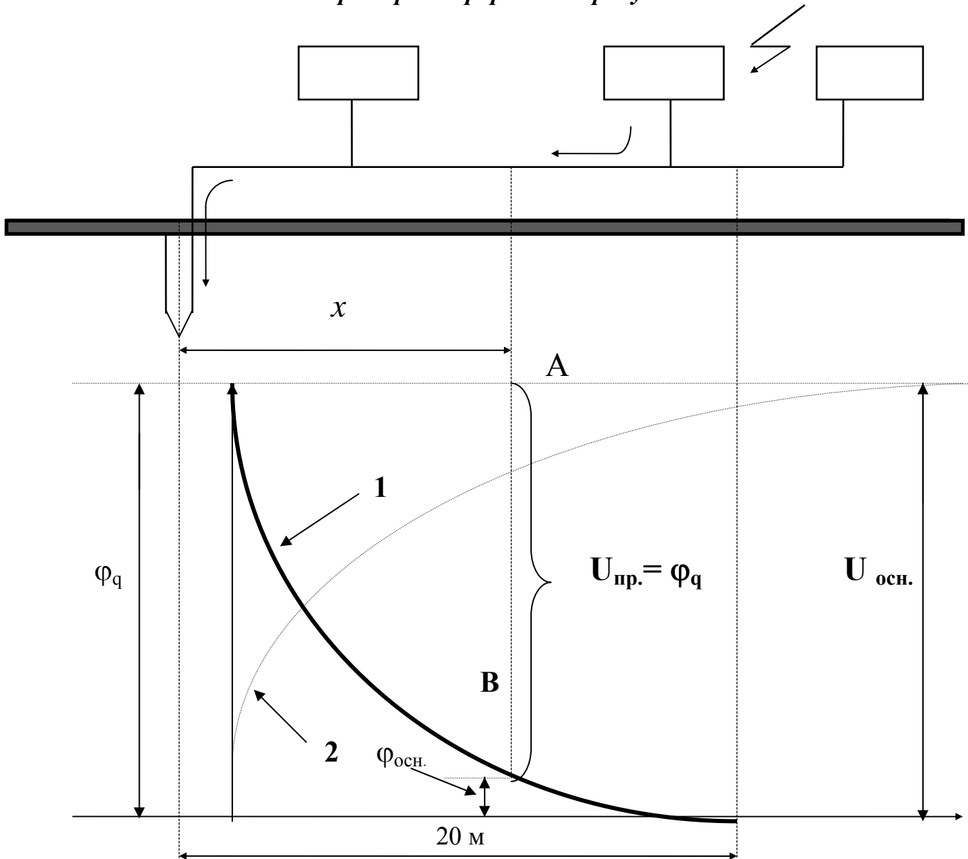
Рисунок 3 – Напряжение прикосновения при одиночном заземлителе: 1 – потенциальная кривая; 2 – кривая, характеризующая изменение U_{пр} при изменении x .
